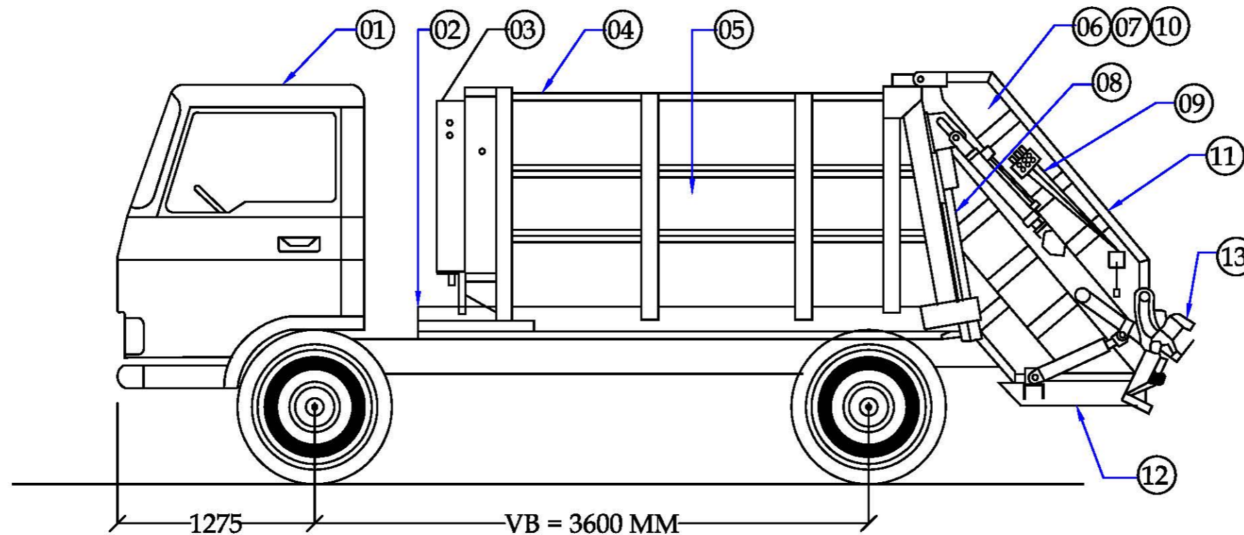
ELEVATION
