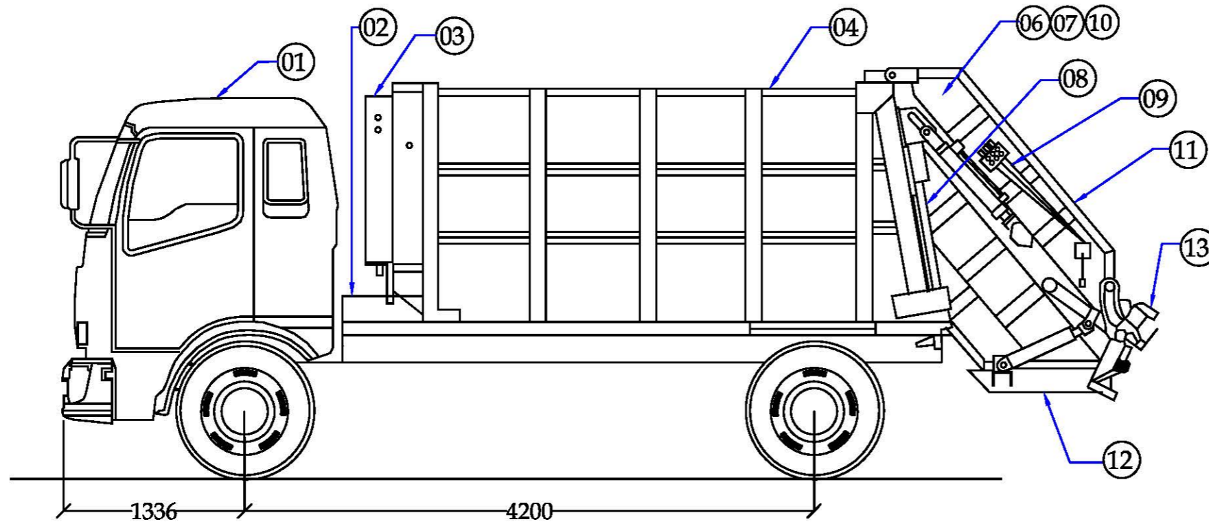
ELEVATION
